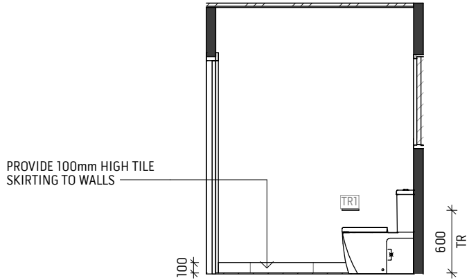
2 A-05-05/ UPPER TOILET 1 SCALE 1 : 50
