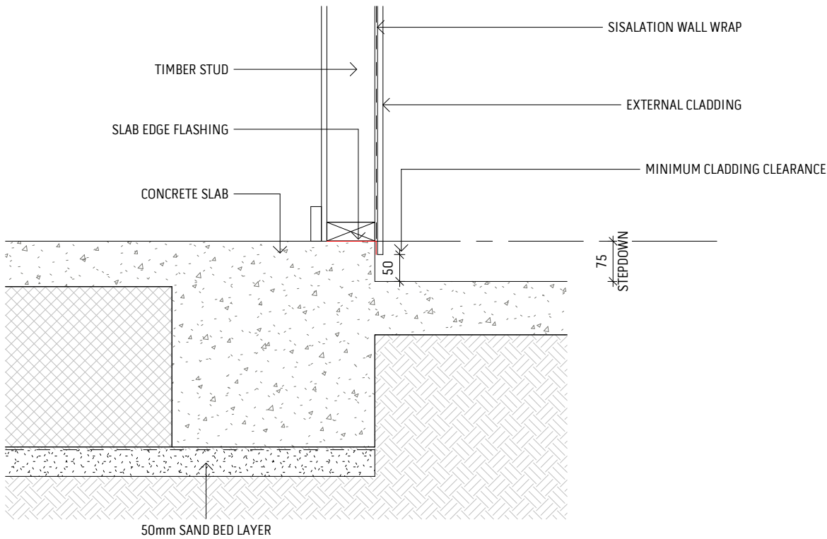
SLAB EDGE DETAIL - ALFRESCO
