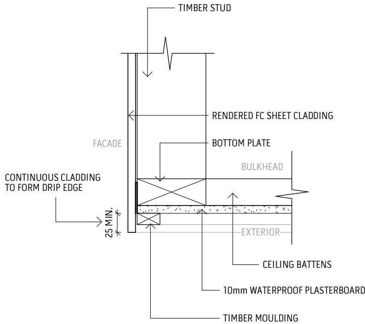
DRIP EDGE DETAIL
