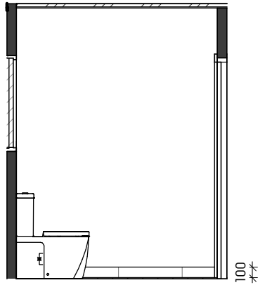
4 A-05-05/ UPPER TOILET 3 SCALE 1 : 50
