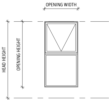
AWNING-FIXED - AF
