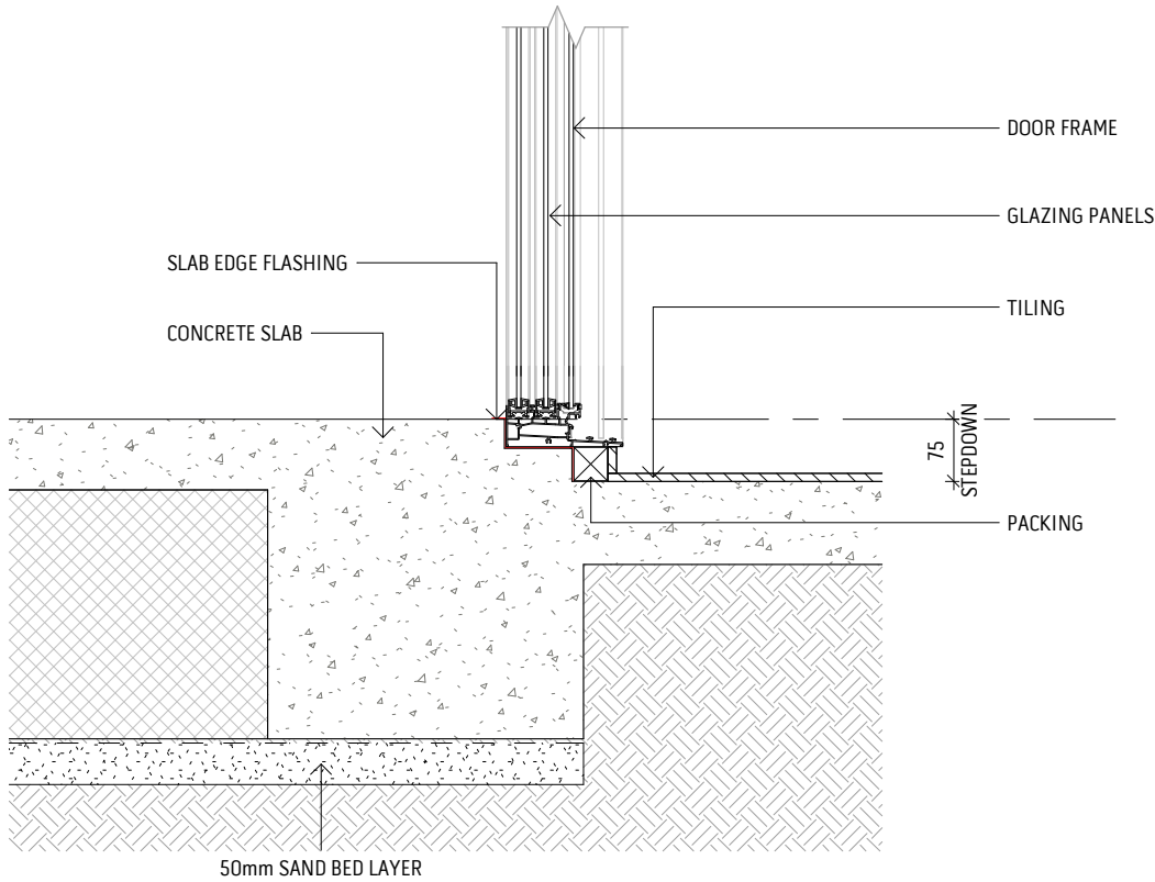
1 / ALFRESCO SLIDING DOOR - DETAIL SCALE 1 : 10
