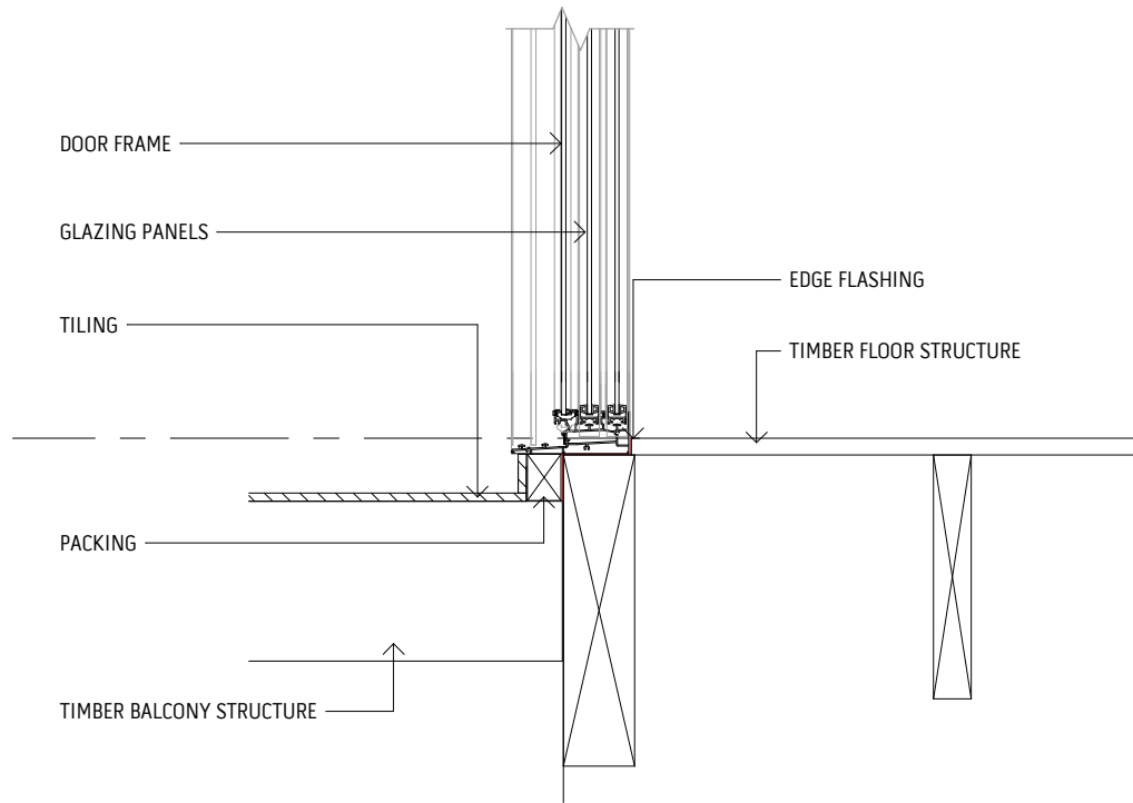
3 / BALCONY SLIDING DOOR - DETAIL SCALE 1 : 10
