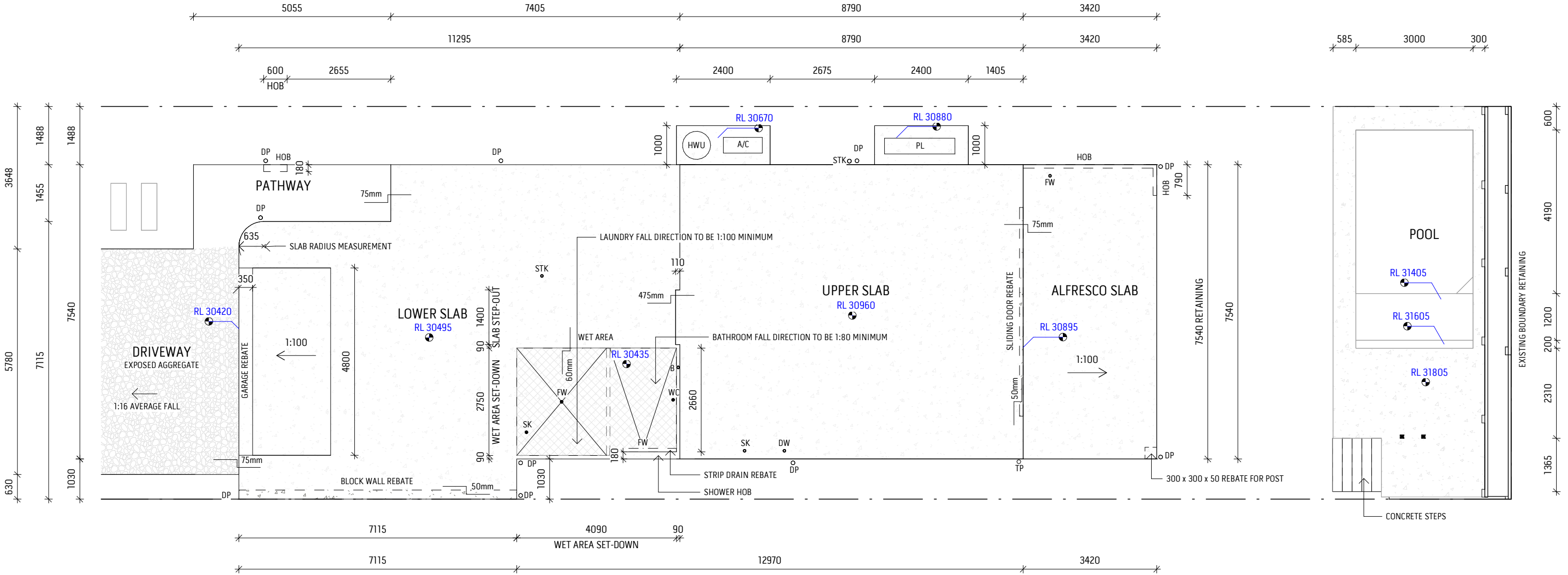
1 A-03-01/ SLAB SETOUT SCALE 1 : 100
