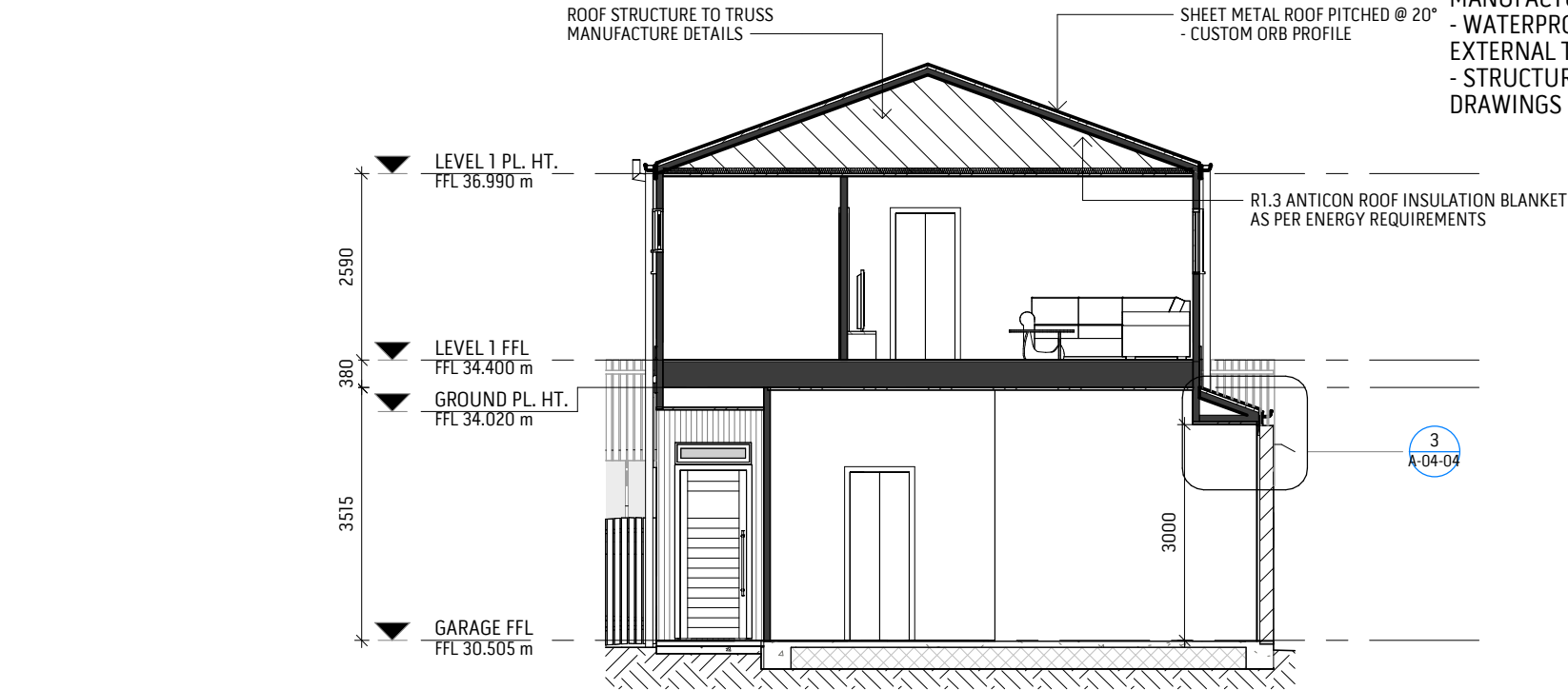
1 A-02-01 SECTION C SCALE 1 : 100
