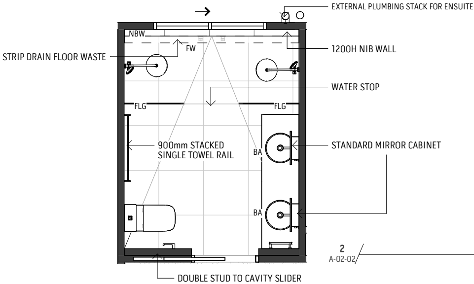
ENSUITE - CALLOUT
