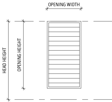
LOUVRE - L
